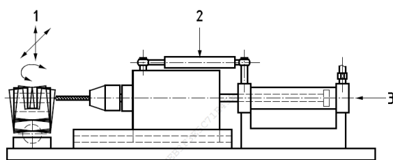
Obrázok 7 Prípravok na skúšanie odolnosti proti odvrtnutiu (STN EN 1629, 2012)
